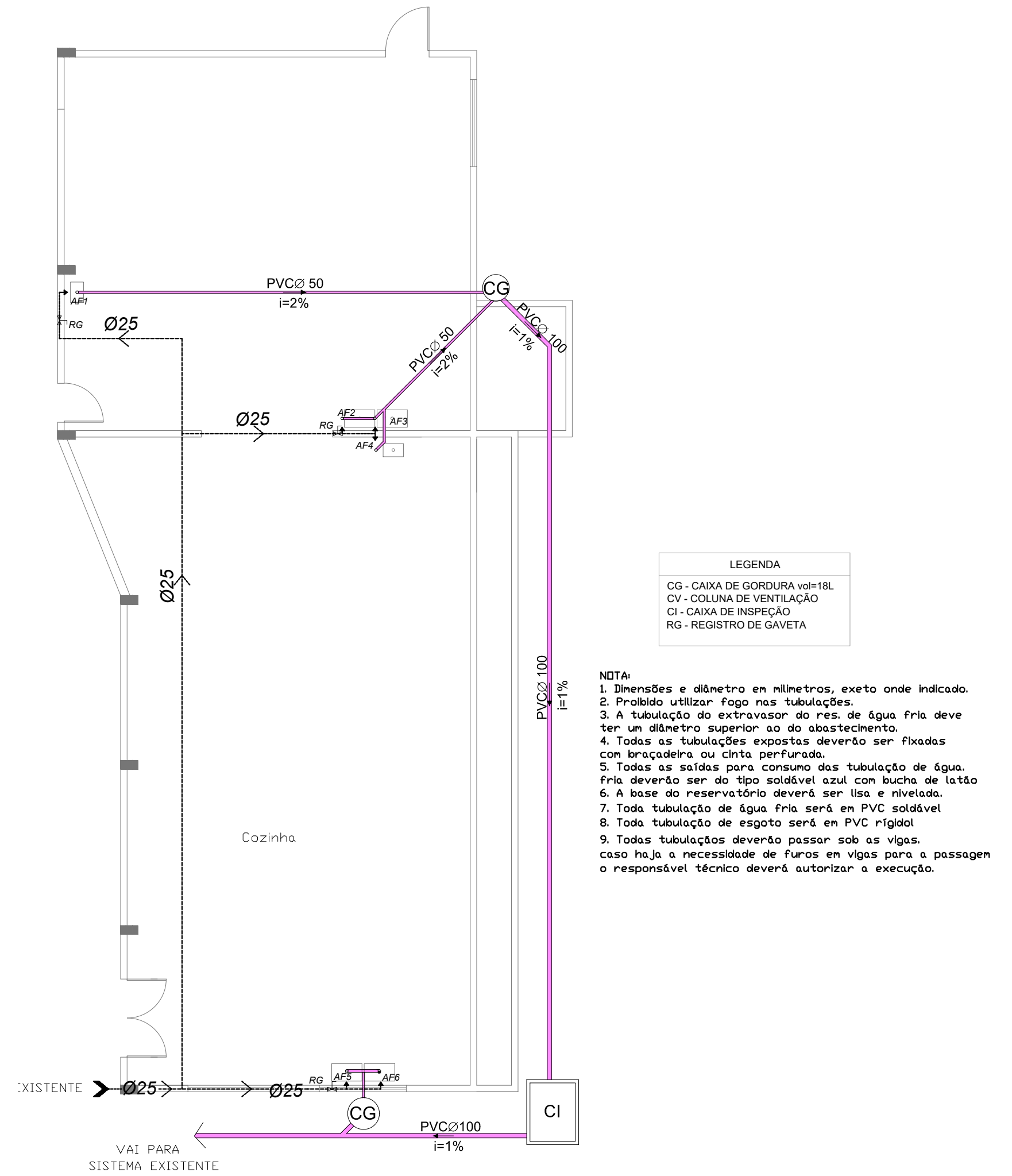
Projeto Hidrossanitário Esc: 1/100
