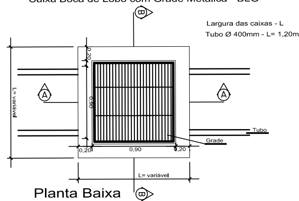
Caixa Boca de Lobo com Grade Metálica - BLG
