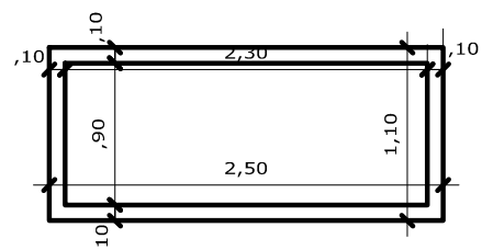
2 PLANTA BAIXA CARNEIRA ADULTO 1:50
